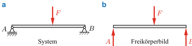
Abb. 1.7 System und Freikörperbild
