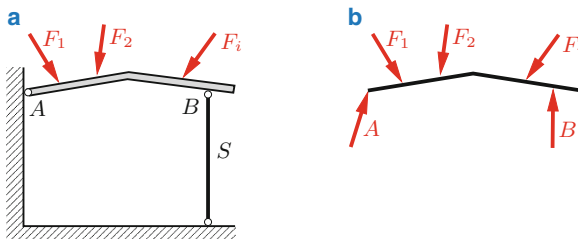
Abb. 5.1 a Tragwerk, b Freikörperbild
