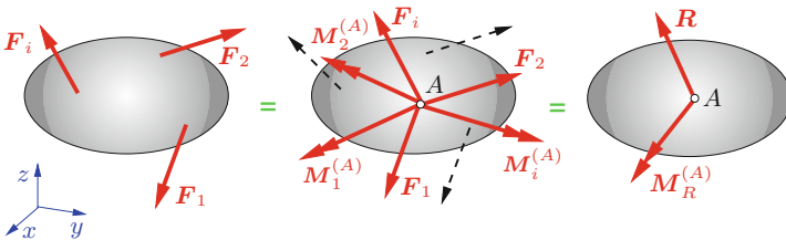
Abb. 3.22 Reduktion eines allgemeinen Kräftesystems im Raum
